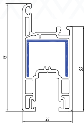
OPS-SF-02 Sliding Door Sash
