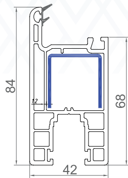
BLS-SF-03 Sliding Door Sash
